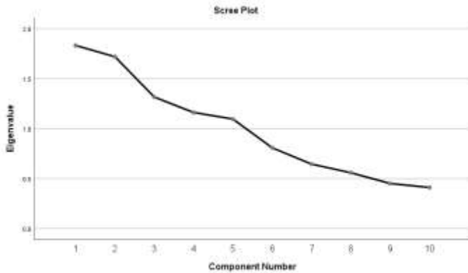
ප්‍රස්තාර සටහන 1: අයිගන් අගයන් සහ සාධක අගයන් (PCF and Varimax)
